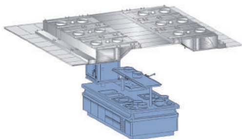
Sufty wentylacyjne
