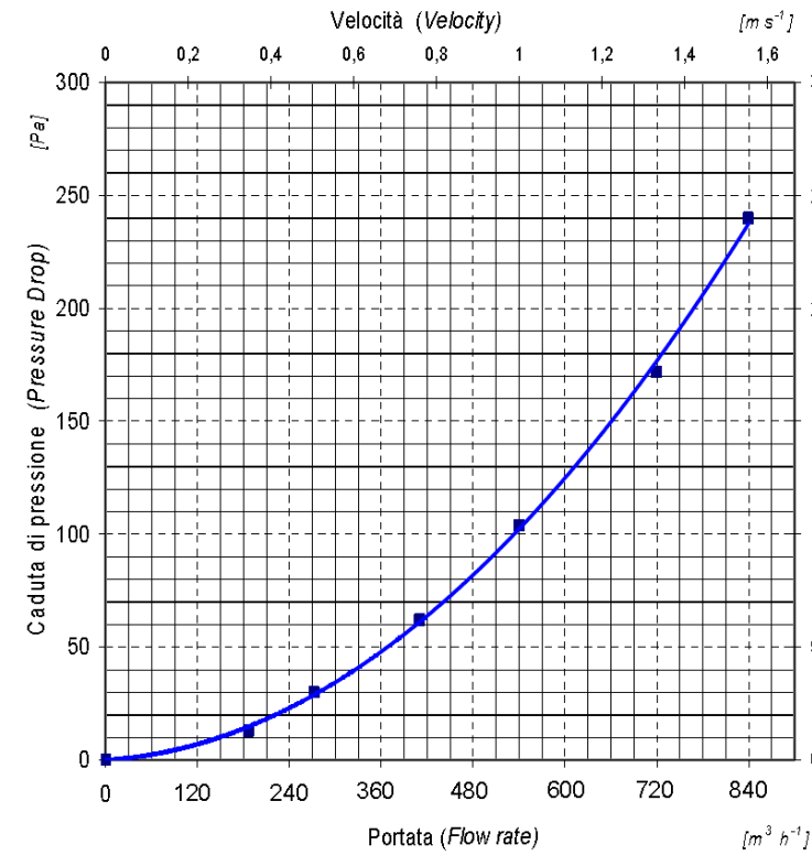
Wykres strat ciśnienia filtra 300x500x20
