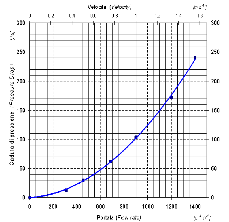
Wykres strat ciśnienia filtra 500x500x20
